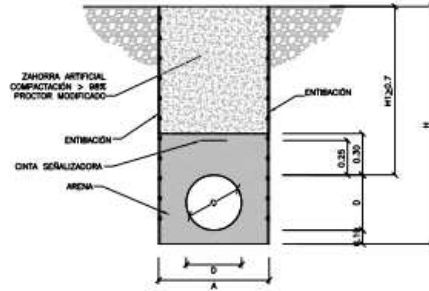
ZANJA EN CAMINO O BERMA
