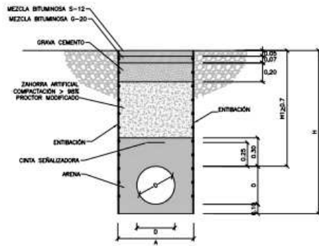
ZANJA EN CARRETERA
