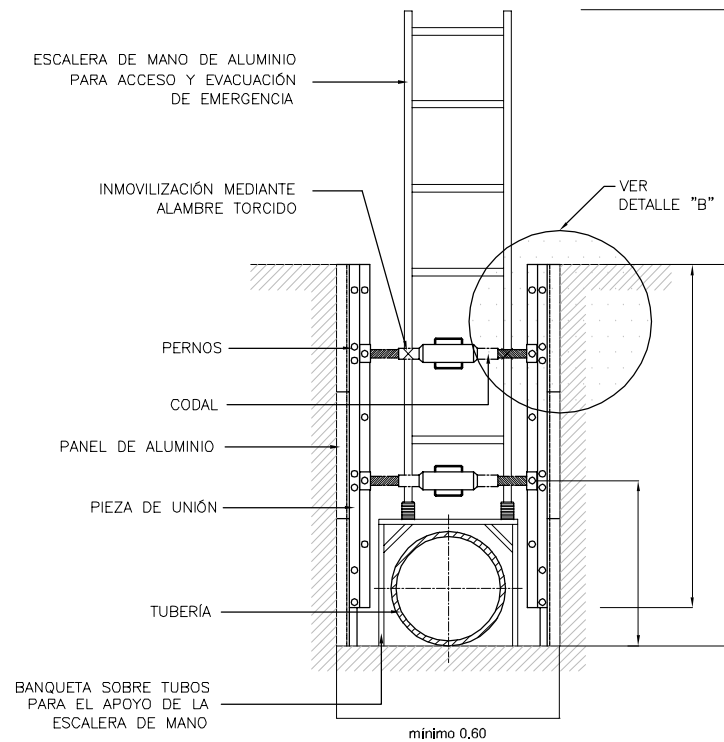
SECCIÓN ESCALA 1/25
