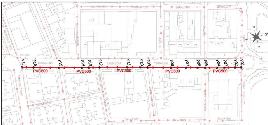
Red de alcantarillado proyectada
