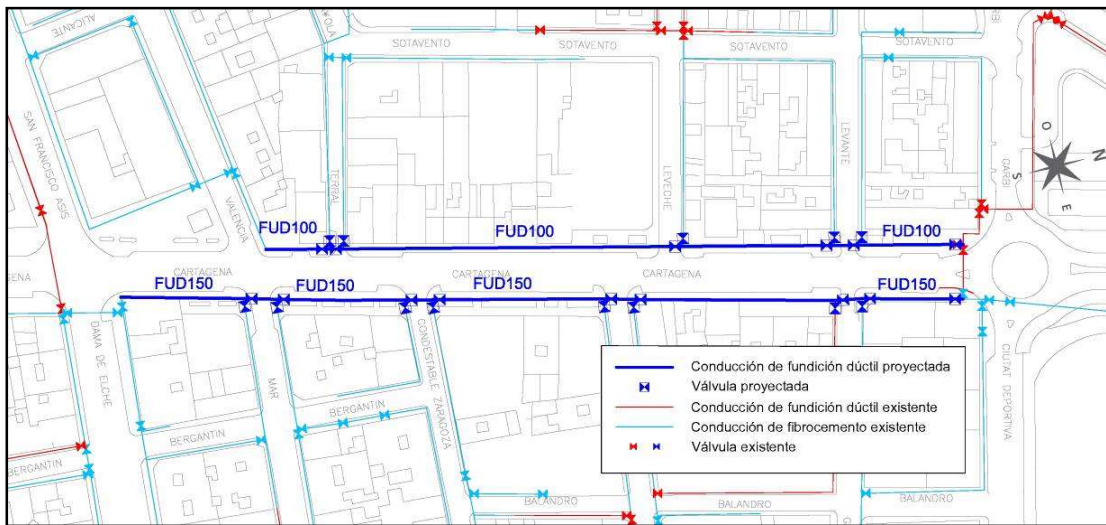
Tuberías de agua potable a instalar
