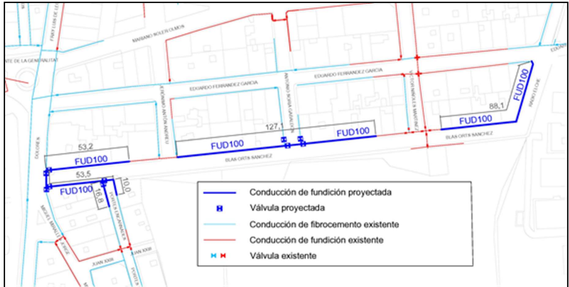
Tramos de tubería de agua potable a instalar
