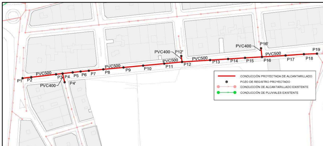
Red de alcantarillado proyectada
