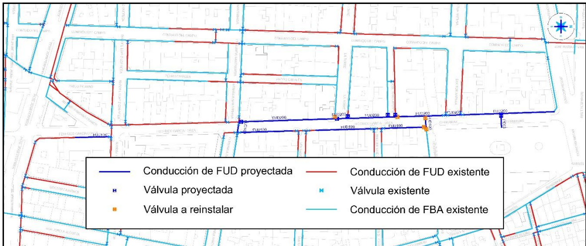
Tramos de tubería de agua potable a instalar
