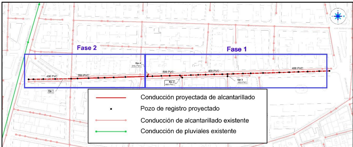
Red de alcantarillado proyectada
