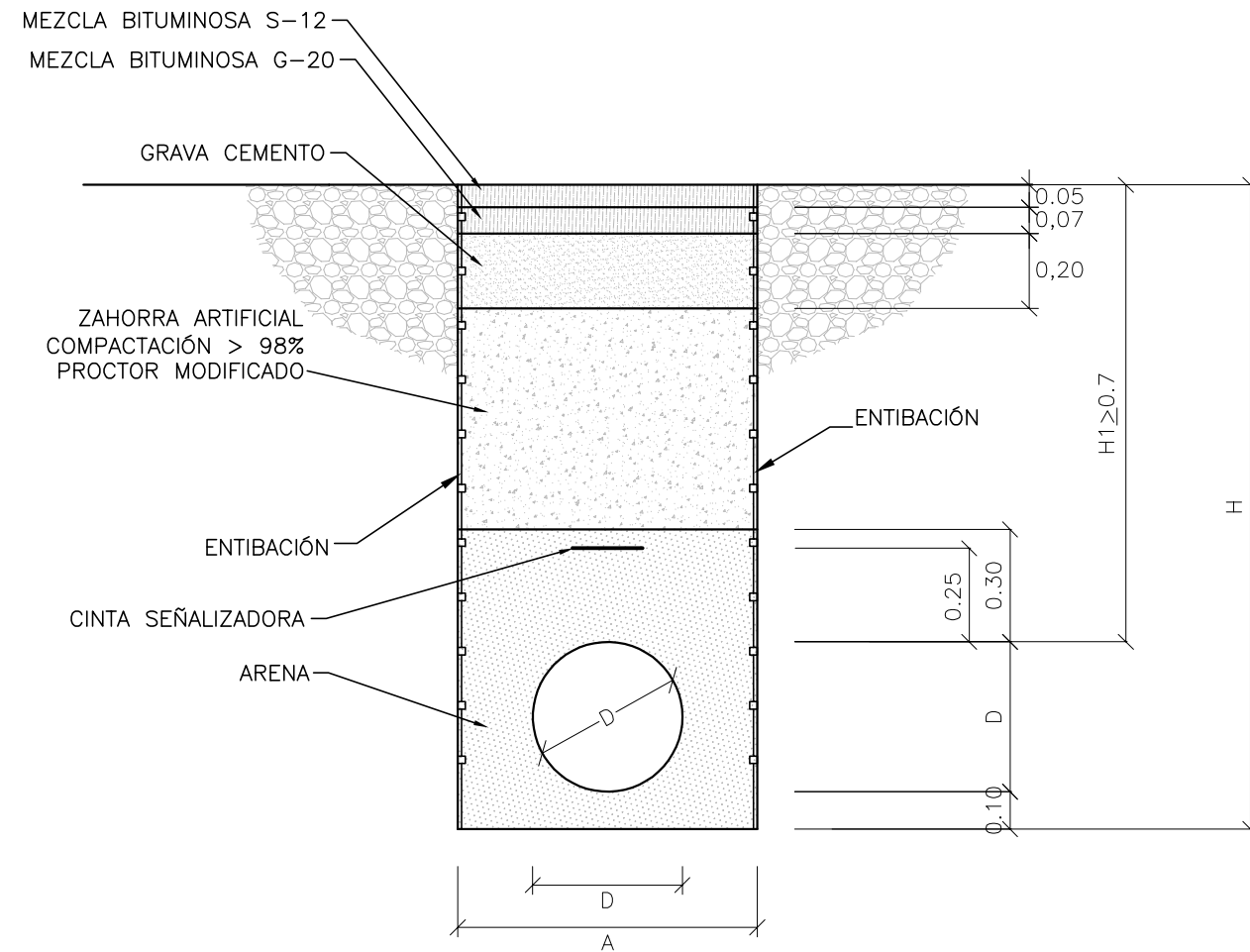
ZANJA EN CARRETERA
