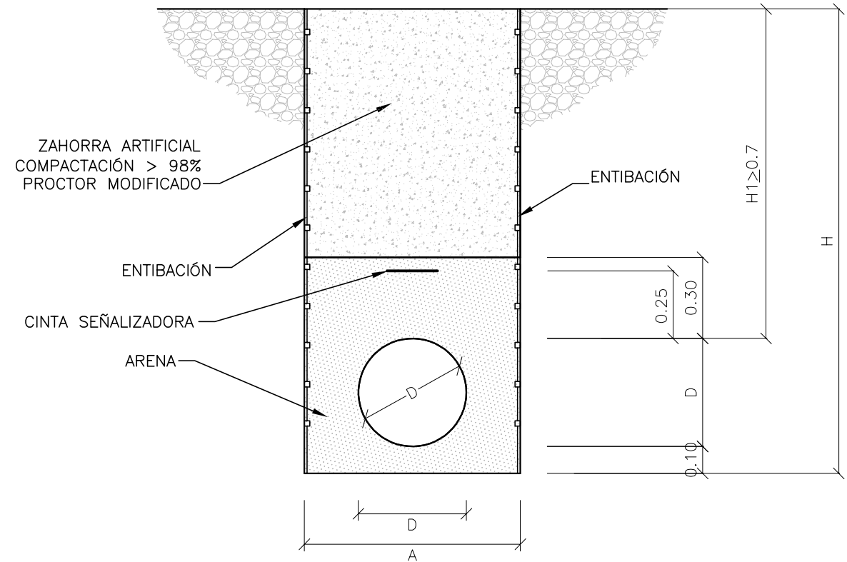
ZANJA EN CAMINO O BERMA
