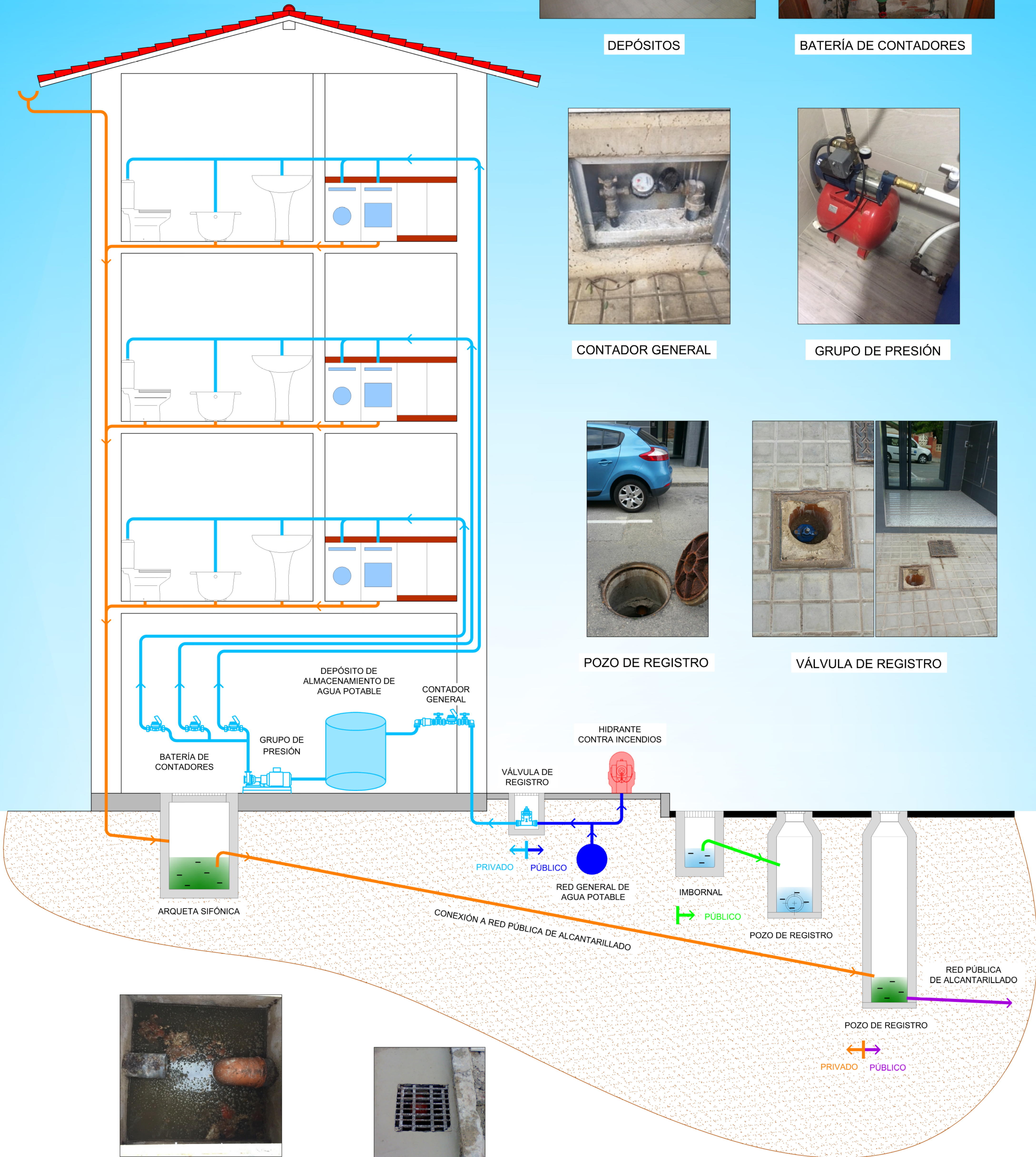
ARQUETA SIFÓNICA
